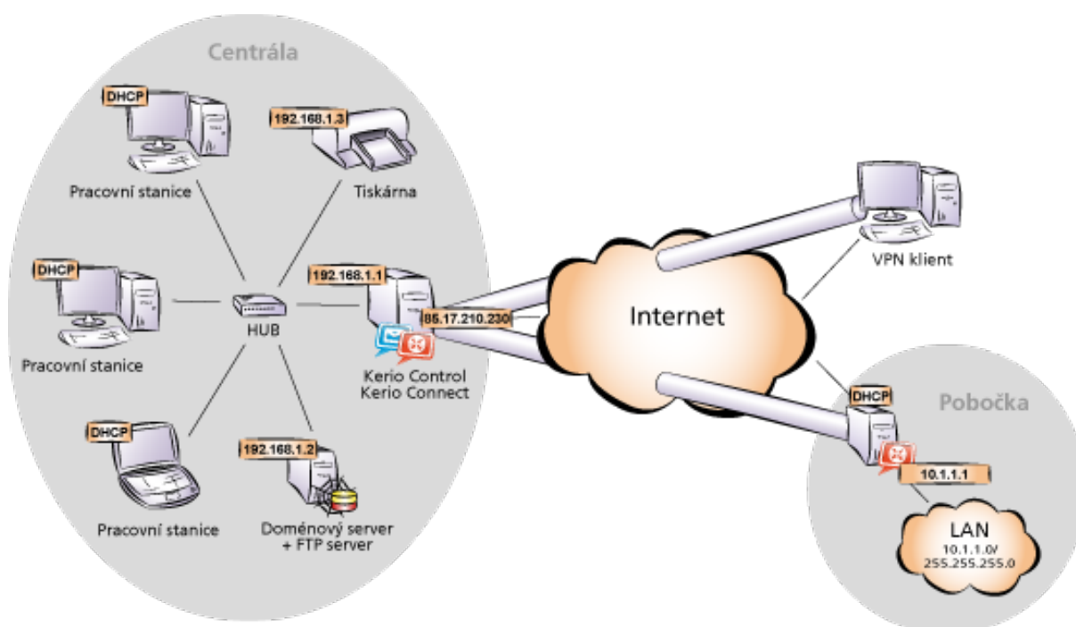
Obrázek 2.1 Modelová konfigurace sítě s přidělenými IP adresami
