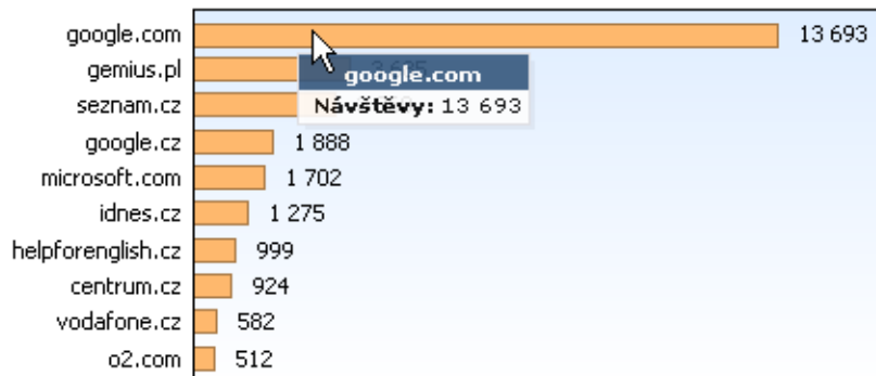
Obrázek 3.20 Nejnavštěvovanější WWW domény
